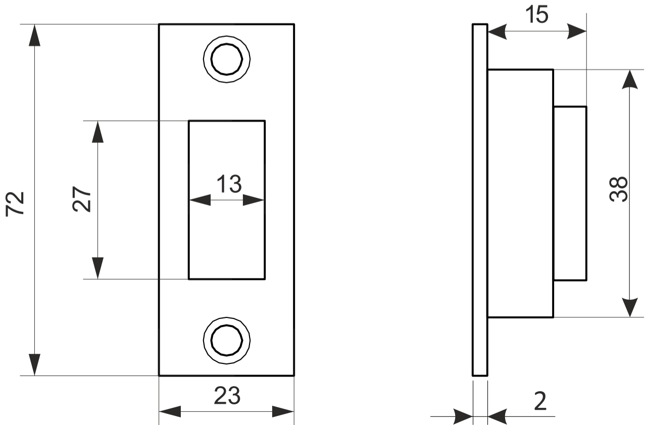
Ответная планка
